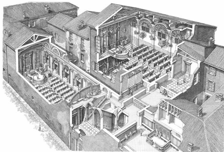
Spaccato assonometrico del complesso di via Mazzini 95 a Ferrara disegno di Francesco Corni su ricostruzione di Paolo Ravenna
